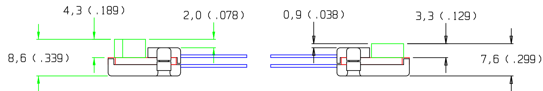
RECEPTACLE QSE
